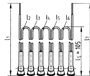
Sechslingsverschaltung
