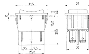
G1/1839.3402 inverseur à impulsion 1-0-1 6(4)A/250V
