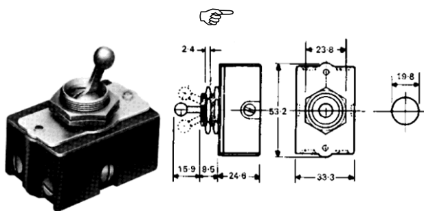
G3/80638-D inverseur avec blocage de commutation au point zéro 5A/250V
