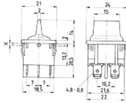
G1/1812.1102 interrupteur 10(4)A/250V G1/1819.1102 inverseur 1-0-1 G1/1819.1302 inverseur à impulsion 1-0-1 6(2)A/250V
