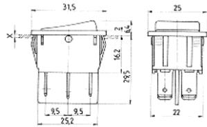
G1/1832.3311 interrupteur blanc G1/1832.3312 interrupteur noir 16(4)A/250V
