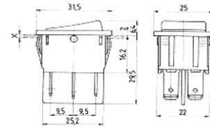
G1/1834.3311 inverseur blanc G1/1834.3312 inverseur noir 16(4)A/250V
