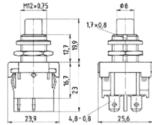
G1/1842.1101 interrupteur G1/1844.1101 inverseur 6(4)A/250V
