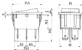
G1/1839.1507 inverseur 1-0-1, noir 6(4)A/250V
