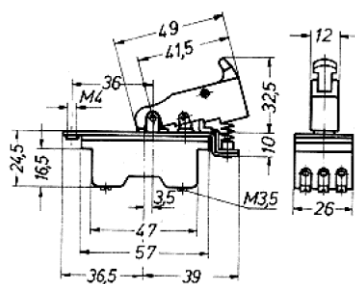
G1/1363.0101 contact de fermeture avec verrouillage 6(6)A/380V
