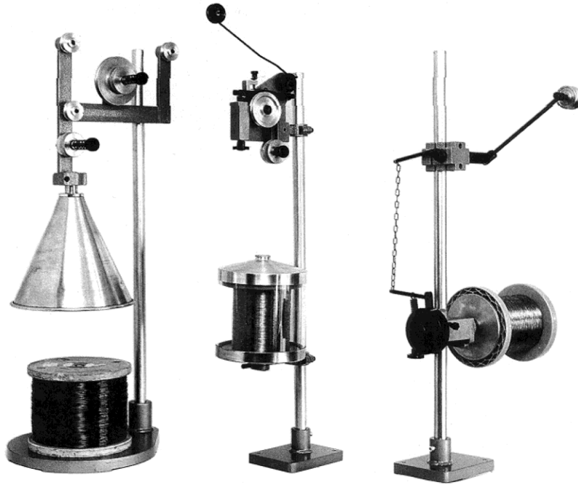
Draht-Ablaufvorrichtungen
