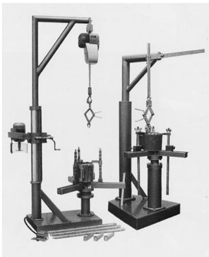
Wickelkopf-Abtrenn- und Ausziehgeräte
