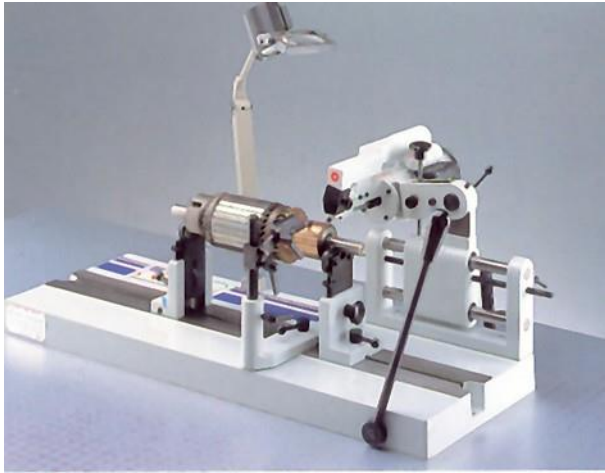
Elektrische Kollektorsägen
