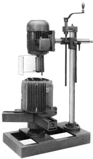
Wickelkopf-Abtrenn- und Ausziehgeräte
