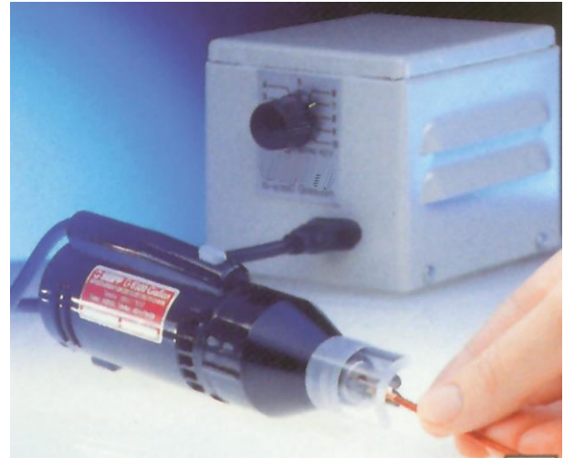
«ABISOFIX»-Abisoliermaschinen für runde Kupferdrähte Typ A01: 0,2 - 0,8 mm Ø Typ A03: 0,6 - 2,0 mm Ø Typ A05: 1,3 - 4,5 mm Ø
