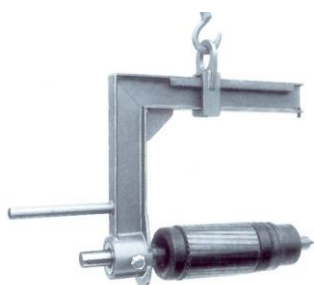
Hebe- und Transport-Vorrichtungen für Anker und Statorn
